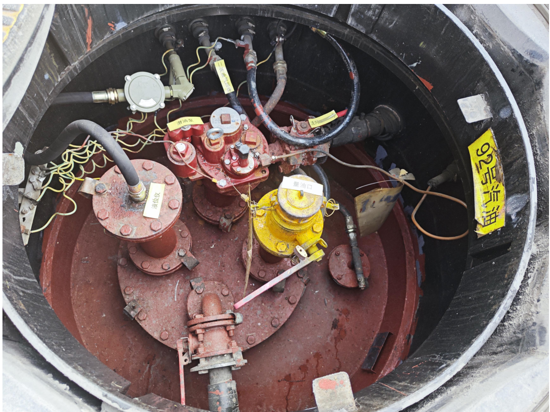
油罐人孔操作井照片
