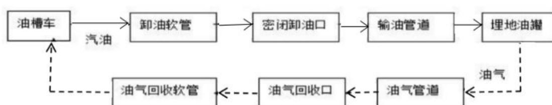
图 2.4-1 汽油卸油工艺流程
