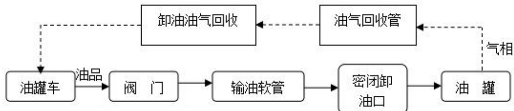
图 2.4-6 汽油卸油工艺及卸油油气回收工艺流程图
