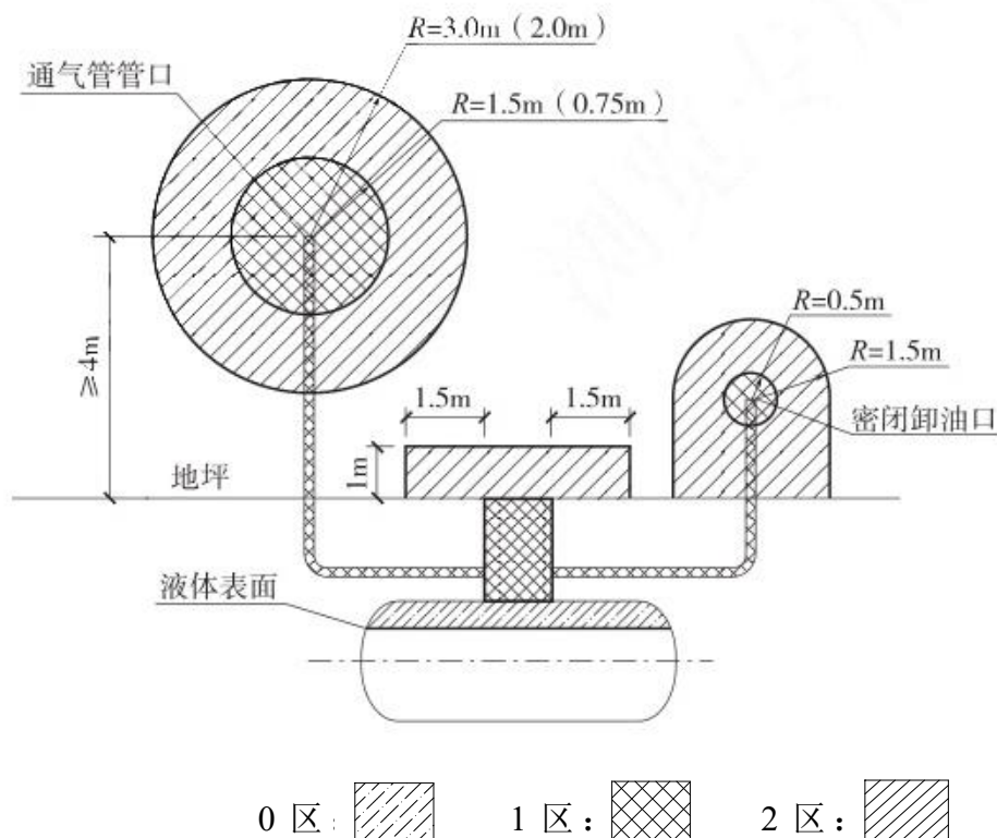
图 3.5-3 汽油埋地卧式油罐的爆炸危险区域划分
