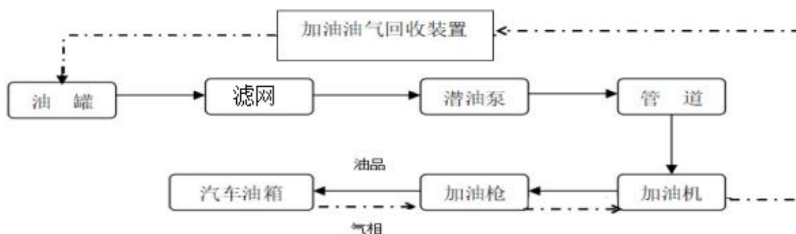
图 2.4-4 汽油加油工艺及加油油气回收工艺流程图
