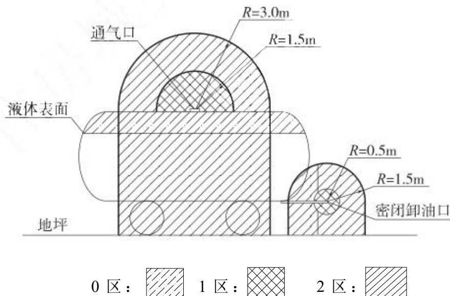
图 3.5-2 汽油油罐车和密闭卸油口的爆炸危险区域划分
