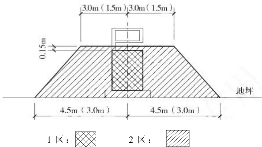
图 3.5-1 汽油加油机的爆炸危险区域划分
