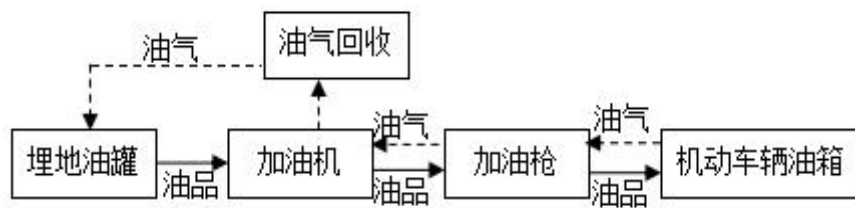
图 2.4-3 汽油加油工艺流程图
