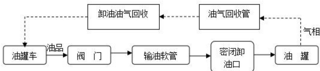
图 2.4-6 汽油卸油油气回收工艺流程图
