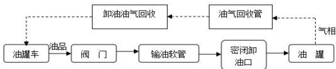
图 2.4-6 汽油卸油油气回收工艺流程图
