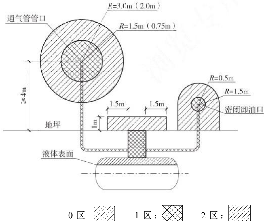
图 3.4-3 汽油埋地卧式油罐的爆炸危险区域划分
