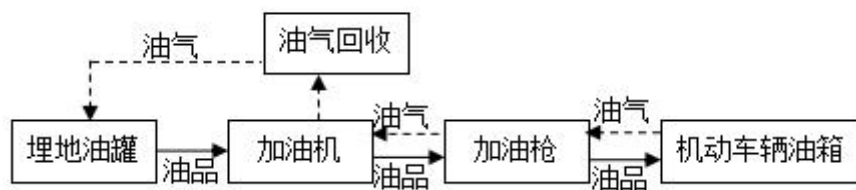
图 2.4-3 汽油加油工艺流程图
