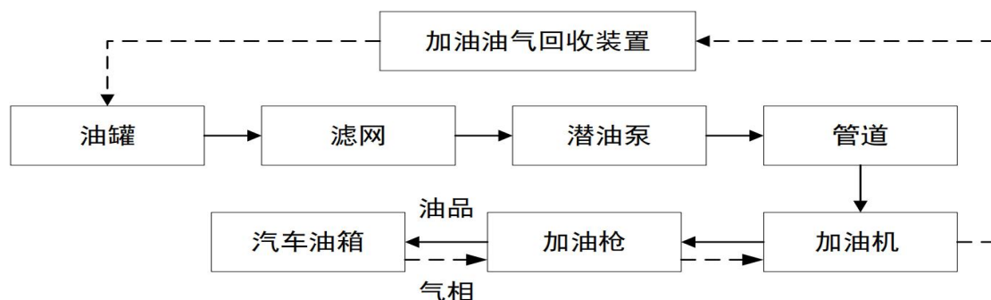
图 2.4-5 汽油加油油气回收工艺流程图
