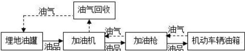
图 2.4-3 汽油加油工艺流程图
