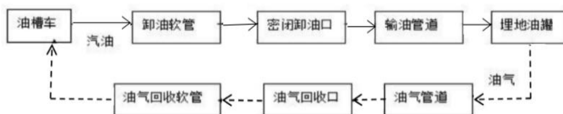
图 2.4-1 汽油卸油工艺流程
