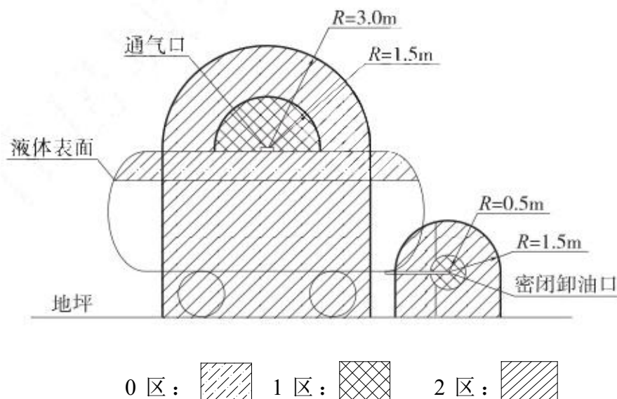
图 3.4-2 汽油油罐车和密闭卸油口的爆炸危险区域划分
