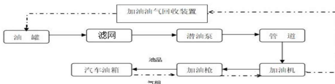
图 2.4-5 汽油加油工艺及加油油气回收工艺流程图
