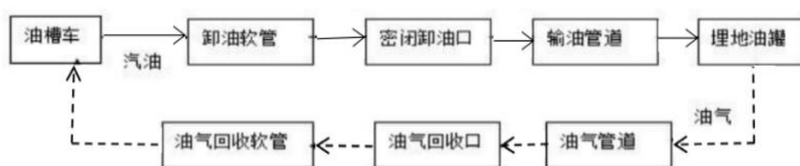
图 2.4-1 汽油卸油工艺流程
