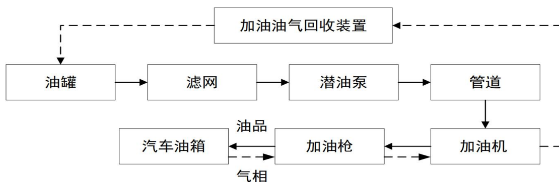
图 2.4-5 汽油加油工艺及加油油气回收工艺流程图
