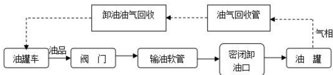
图 2.4-6 汽油卸油工艺及卸油油气回收工艺流程图
