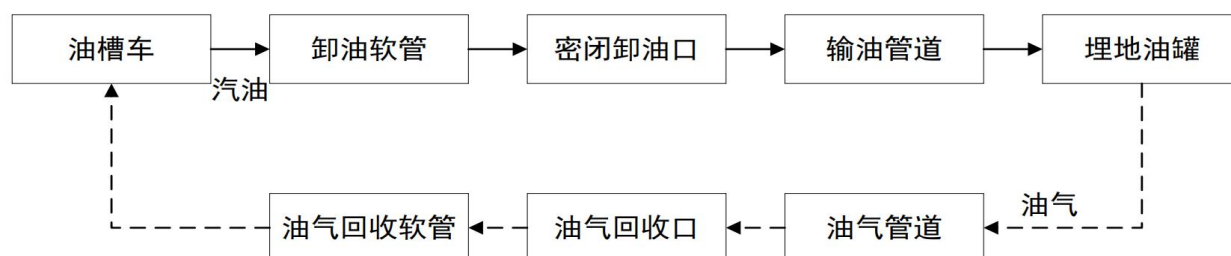
图 2.4-1 汽油卸油工艺流程
