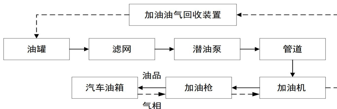
图 2.4-5 汽油加油工艺及加油油气回收工艺流程图
