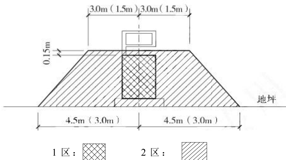
图 3.6-1 汽油加油机的爆炸危险区域划分
