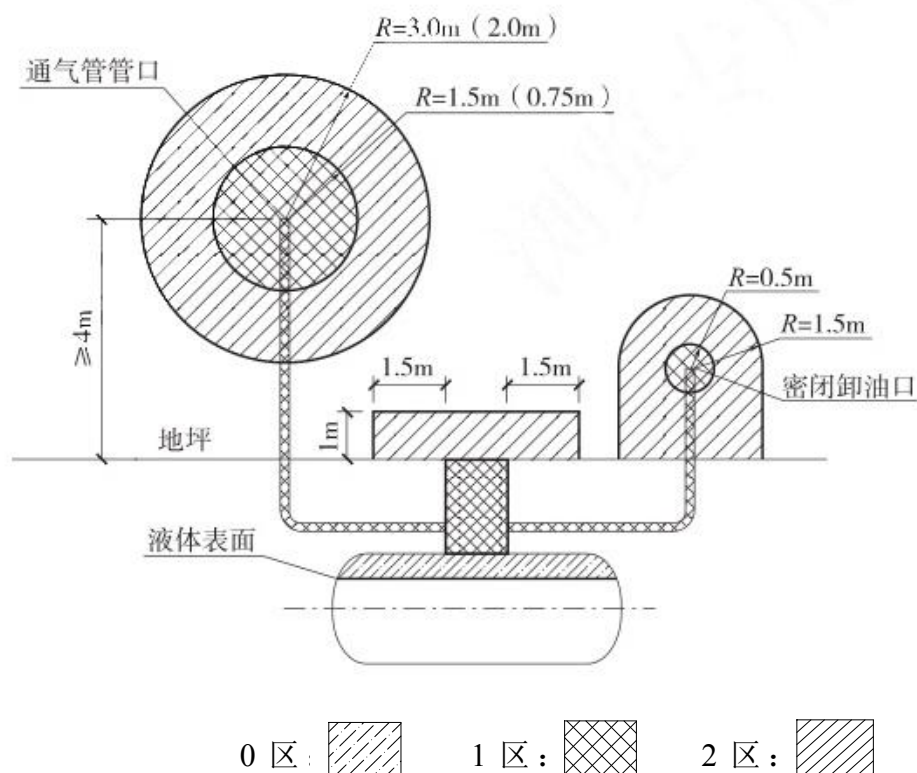
图 3.6-3 汽油埋地卧式油罐的爆炸危险区域划分
