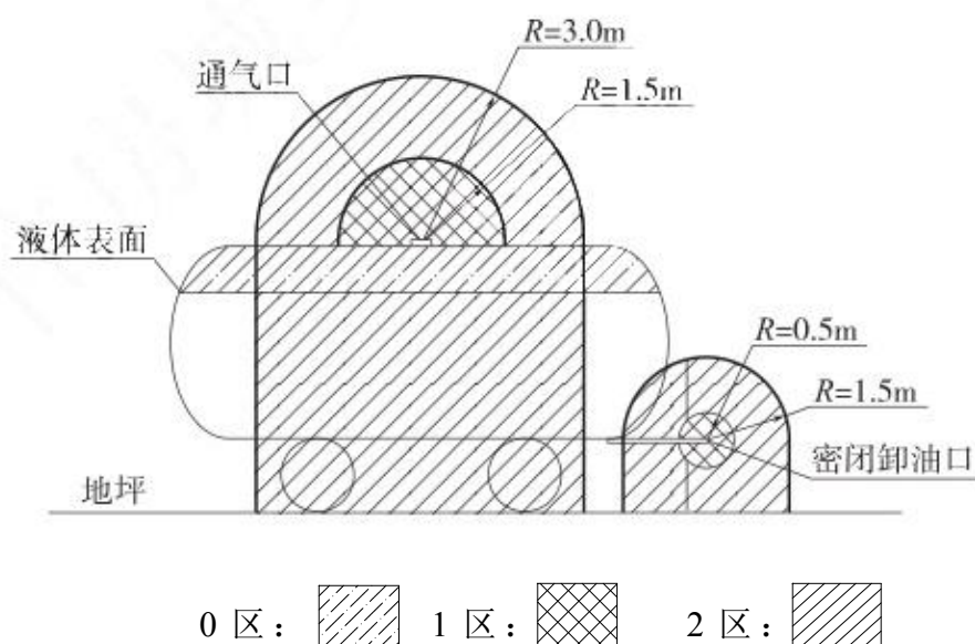
图 3.6-2 汽油油罐车和密闭卸油口的爆炸危险区域划分
