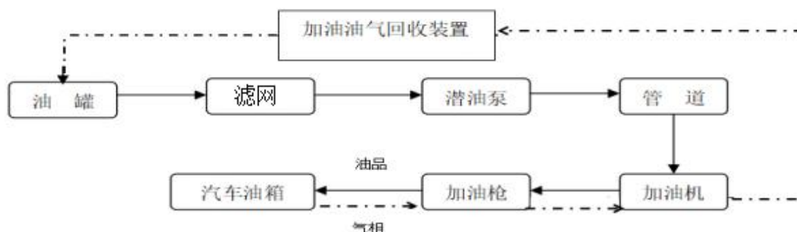
图 2.4-5 汽油加油工艺及加油油气回收工艺流程图
