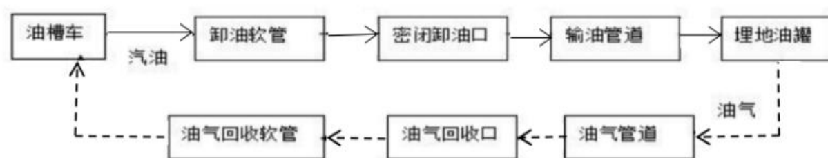
图 2.4-1 卸油工艺流程
