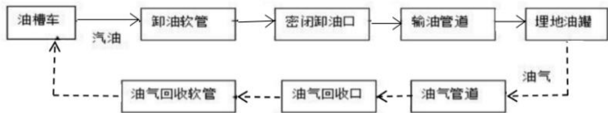
图 2.4-1 卸油工艺流程
